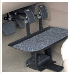
Pedalverlängerung
